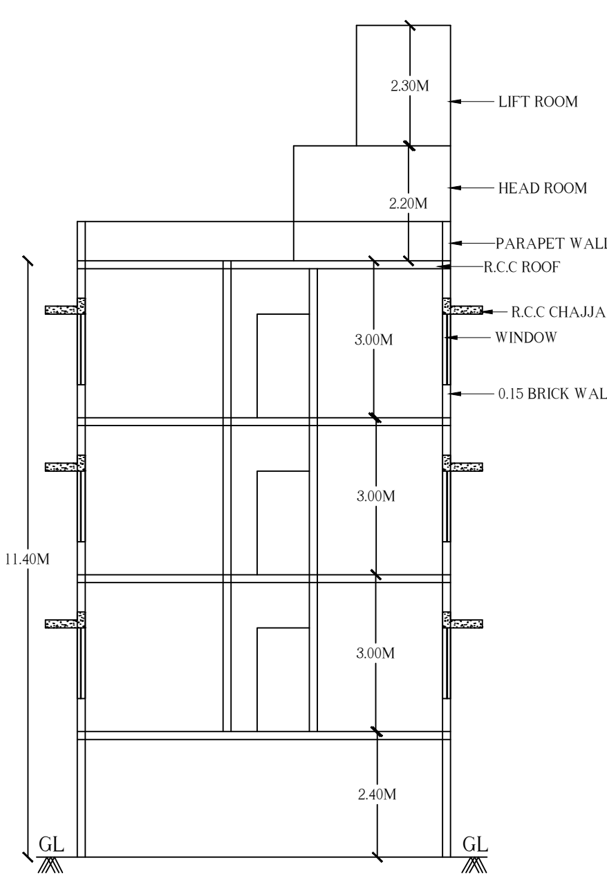
SECTION A-A
